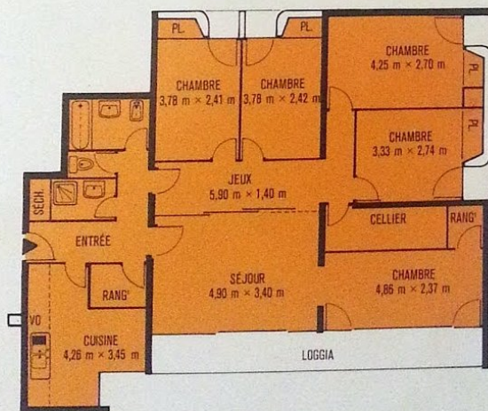
6 pièces type B. 111.60 m 2 + loggia 12.70 m 2
