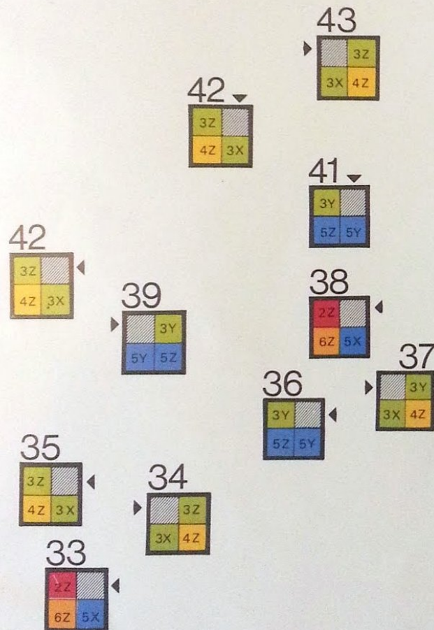
PLAN REZ-DE-CHAUSSÉE
