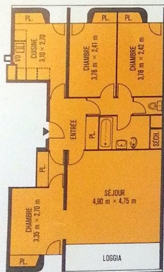
4 pièces type G. 79,40 m 2 + loggia 6,30 m 2 (Le 4 pièces type H est identique quant à la disposition des pièces, mais sa superficie est de 79 m 2 + loggia 6,30 m 2 )
